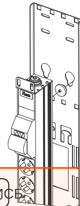
Установка блока розеток на органайзеры с отверстиями для безинструментального монтажа при помощи монтажных шрифтов (только для R-32)
