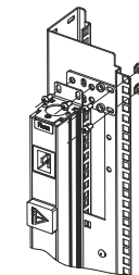
Установка блока розеток на юнитовые направляющие в шкафах ШТК-С-45
