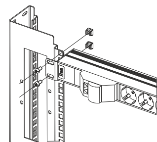
Установка блока розеток на стандартные 19" конструктивы
