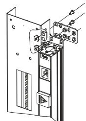
Установка блока розеток в стойки СТК
