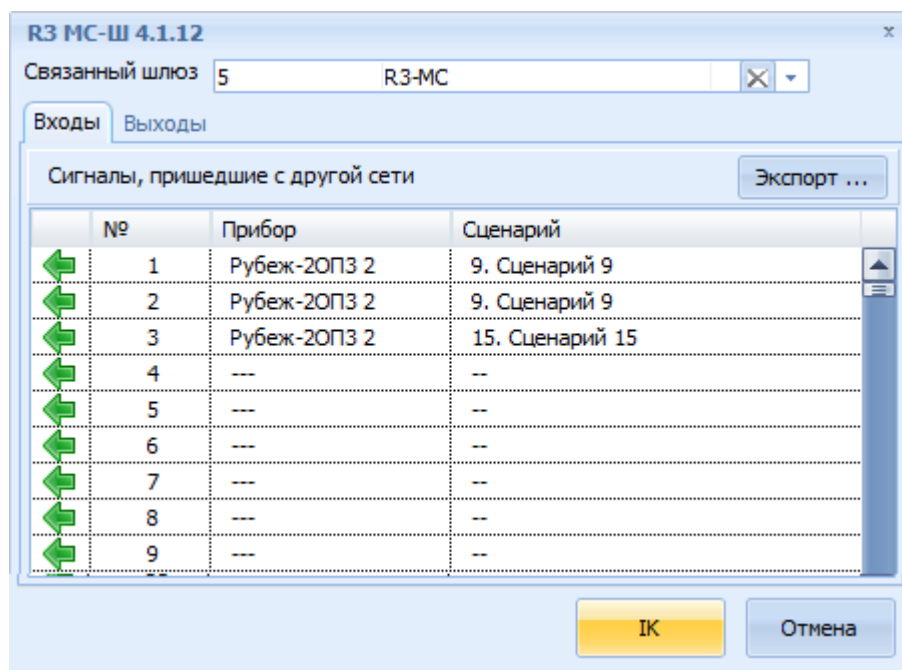
Окно «Свойства R3-MC-Ш»
