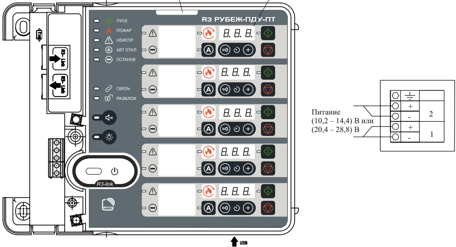
Рисунок 1 – Внешний вид и схема подключения прибора
