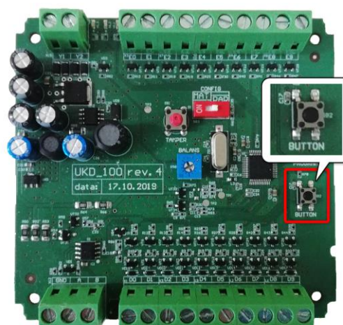
кнопка “ТЕСТ”
