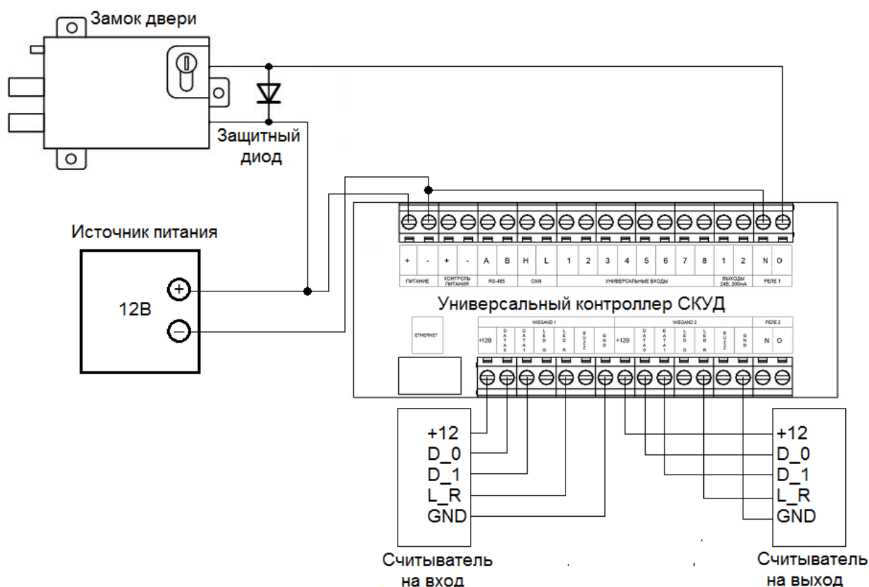
Рисунок 4 – Схема подключения считыватель-считыватель
