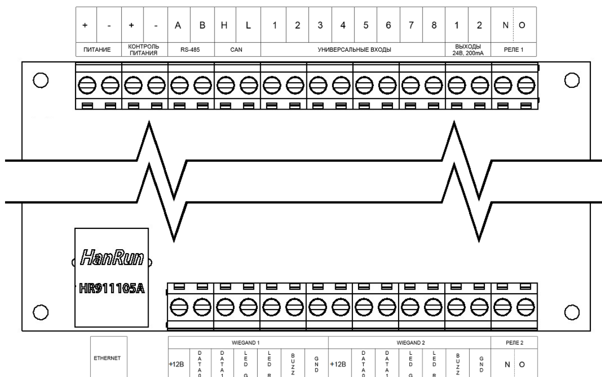
Рисунок 3 – Распиновка клеммных колодок
