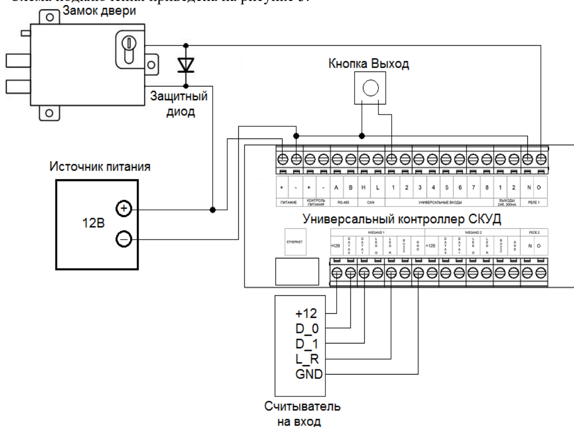
Рисунок 5 - Схема подключения считыватель-кнопка
