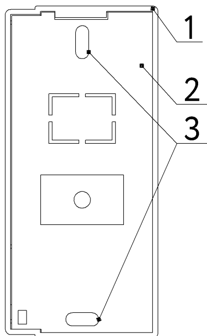
Рисунок 2 – Внешний вид считывателя (сзади)
