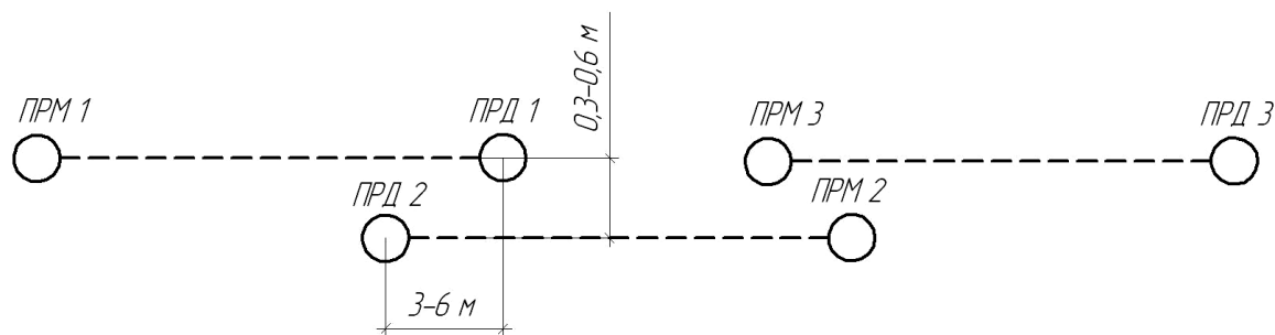
Рисунок 2.1 – Линейное расположение с перекрытием участков
