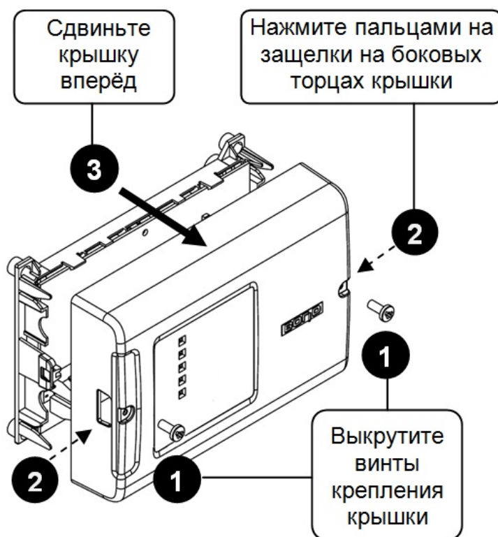
Рисунок 2.2.4.1-1 Снятие крышки
