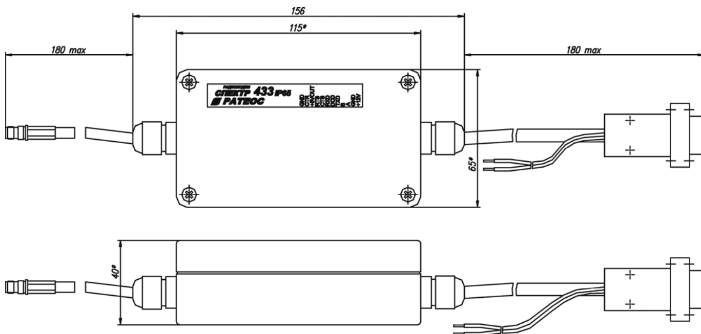
Исполнение IP65
