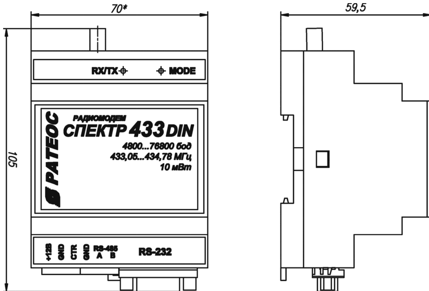
Исполнение DIN
