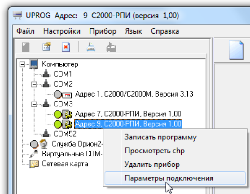
Рисунок 2.2.5.3.3.1 Пункт меню «Параметры подключения»
