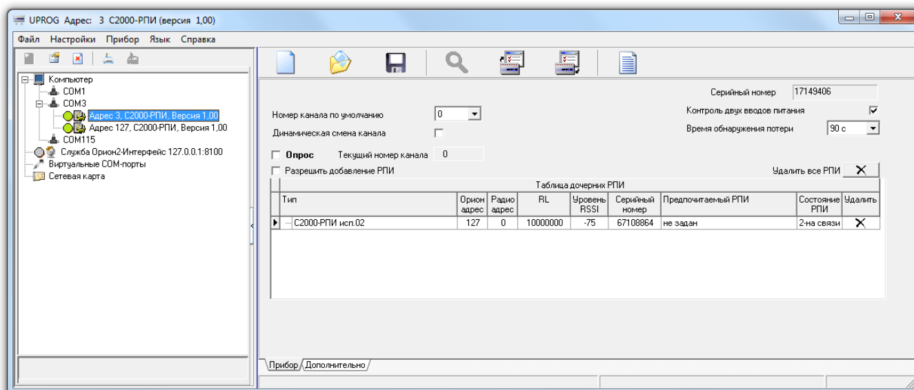
Рисунок 2.2.5.3.2.3 Конфигурация РПИ-мастера
