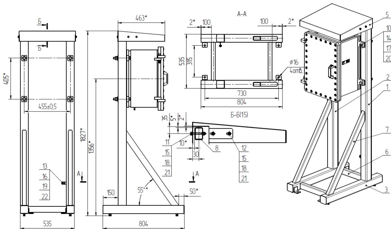
Рис. 2 – Габаритные размеры Спектрон-PM-03
