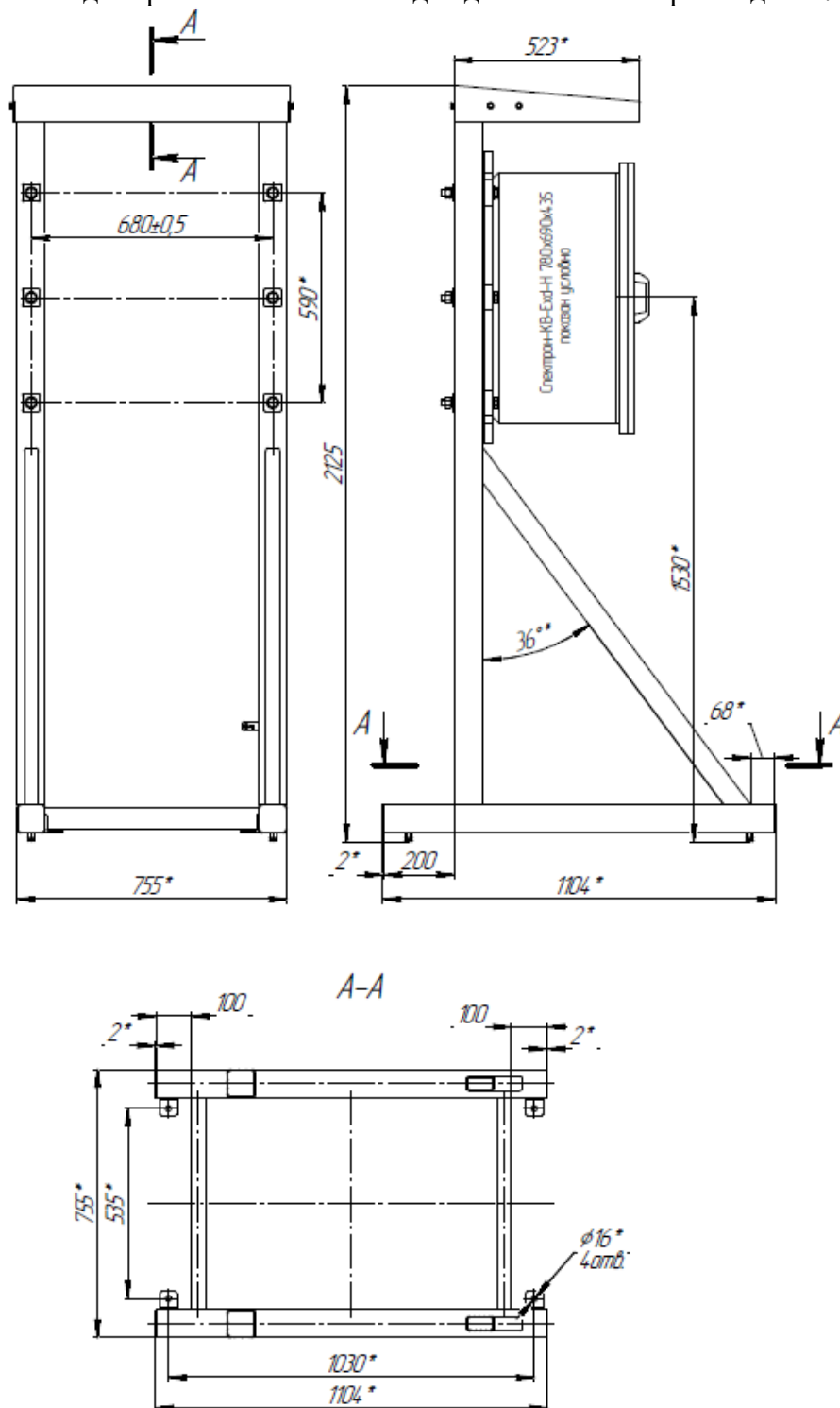
Рис. 1 – Габаритные размеры Спектрон-PM-02
