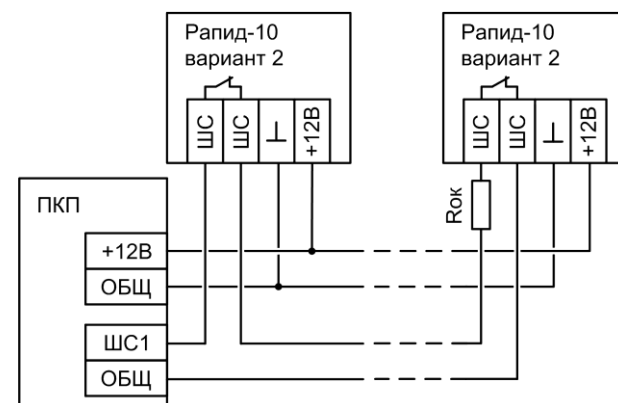
Рис. 2 Схема подключения извещателей к ПКП
