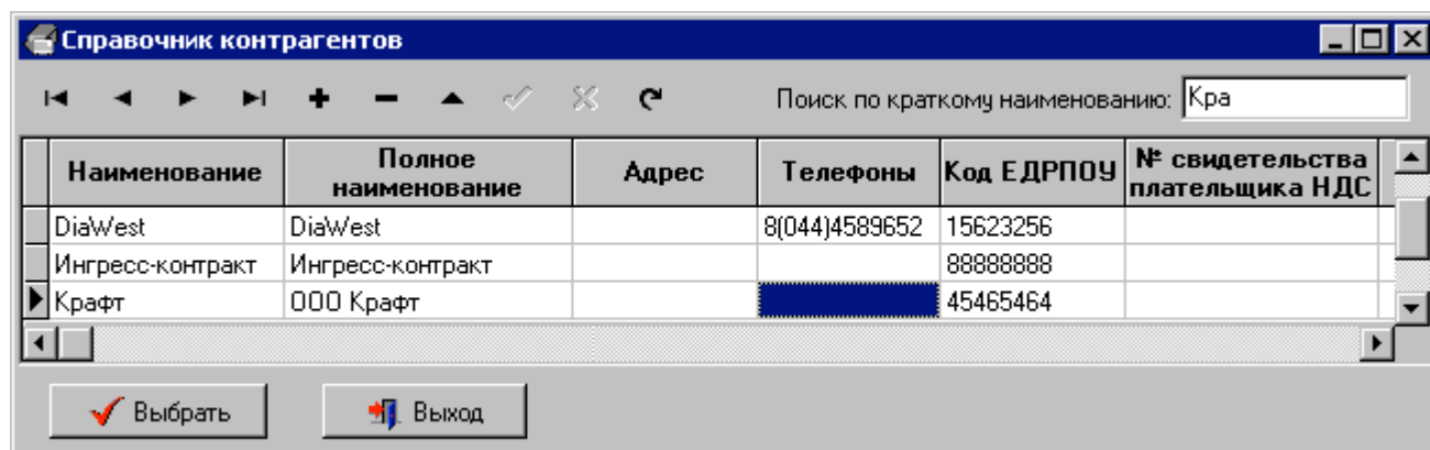
Рис.3.7.1.5. Справочник контрагентов
