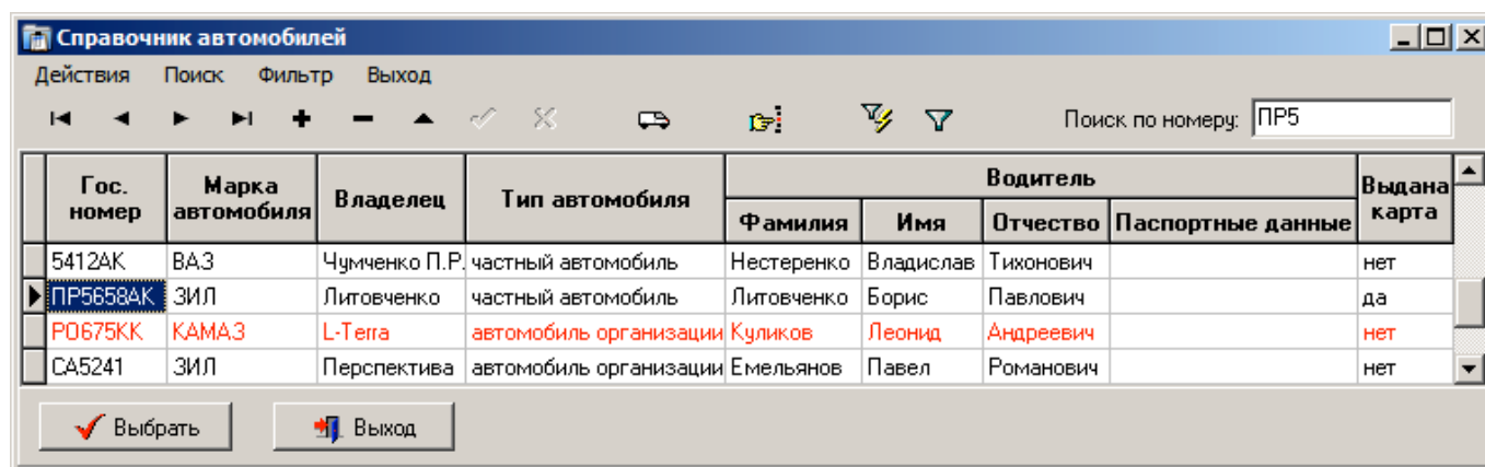
Рис.3.7.1.3. Справочник автомобилей
