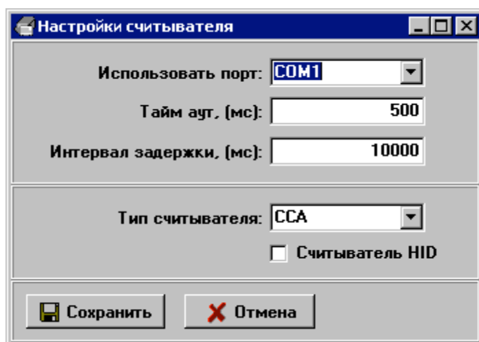
Рис.2.2.1.1. Настройки считывателя
