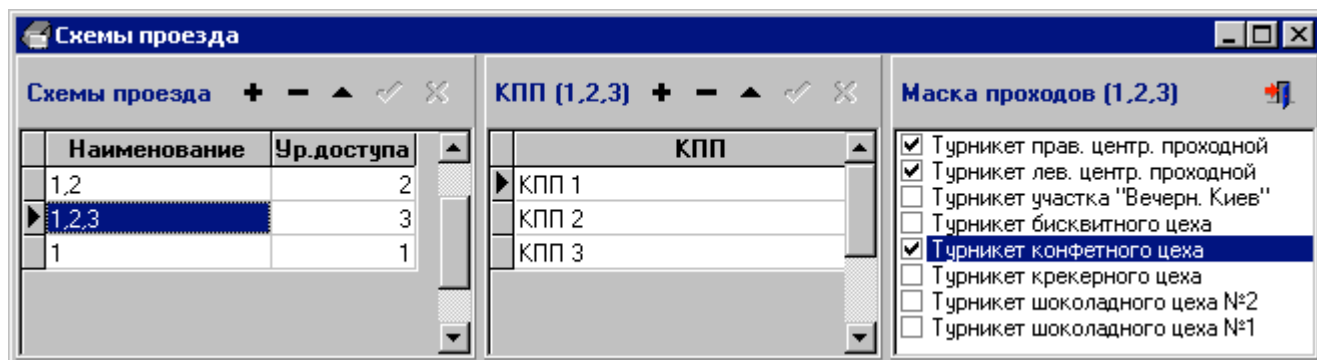
Рис.3.7.1.2. Схемы проезда
