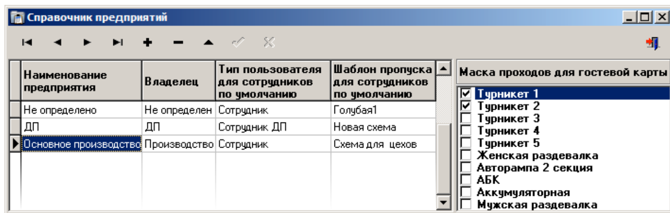
Рис.2.2.4.1. Справочник предприятий
