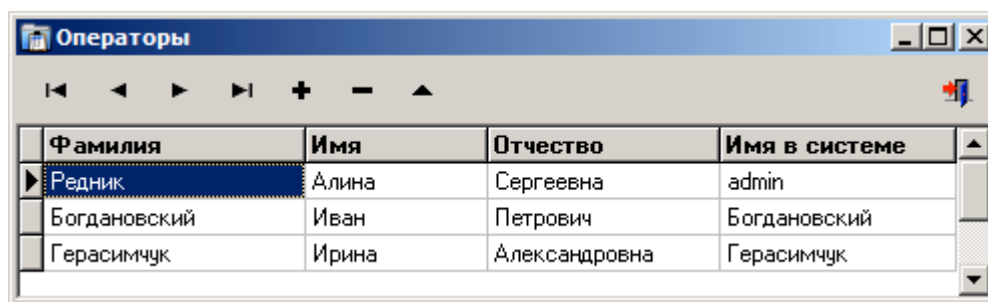
Рис.2.2.5.1. Окно «Операторы»
