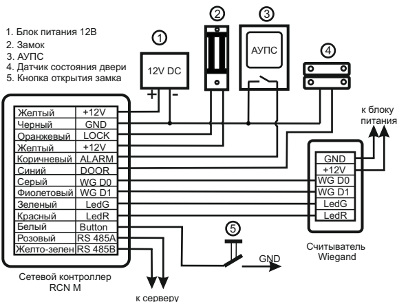
Подключение контроллера «RCN М»
