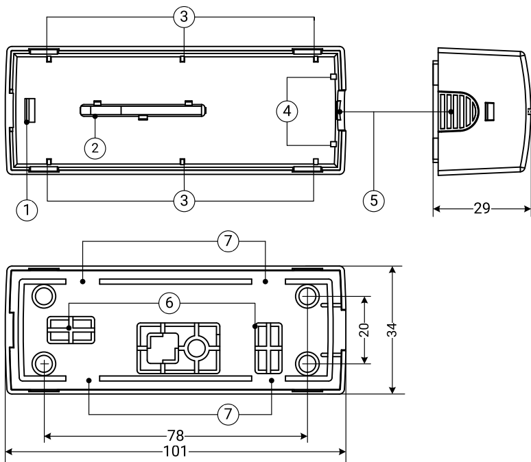
Рисунок 2. Корпус приёмника
