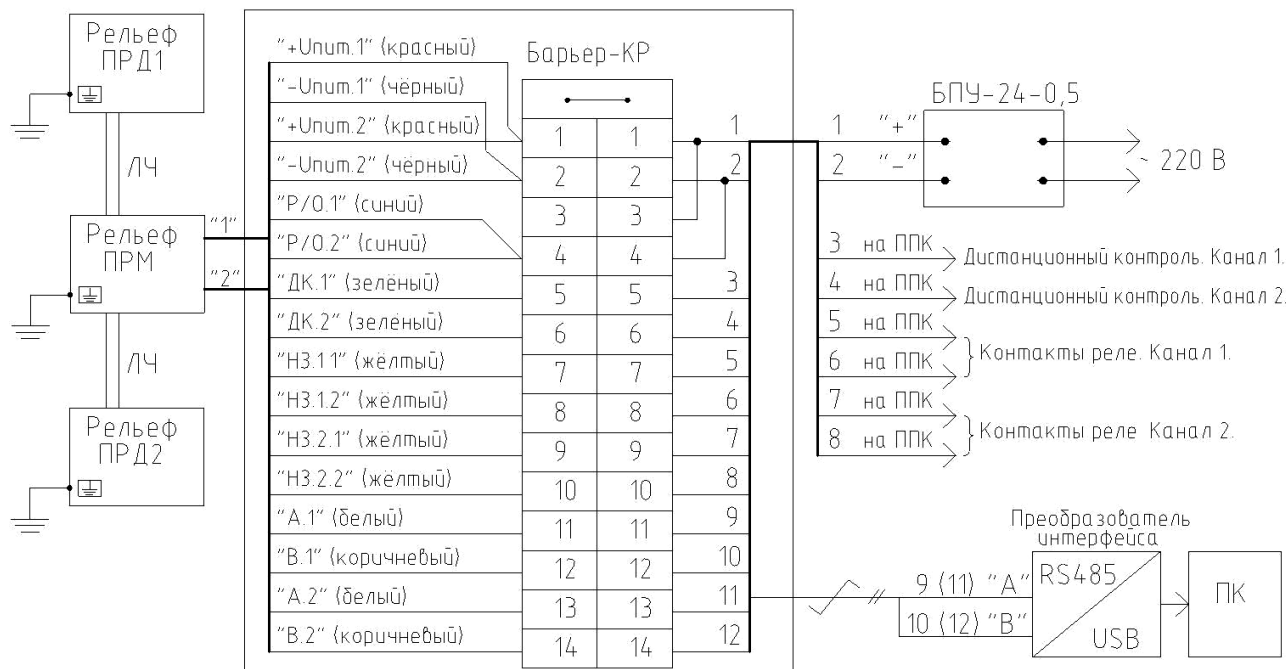
Рисунок 2.9 – Подключение извещателя к коробке распределительной в режиме настройки чувствительности (индикатор выключен).
