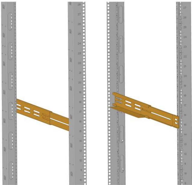
Вид сбоку
