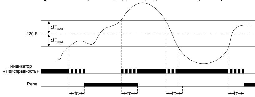
Рисунок 3. Контроль напряжения фазы
