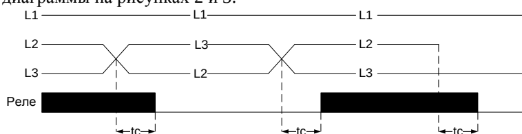
Рисунок 2. Контроль порядка чередования и обрыва фаз
