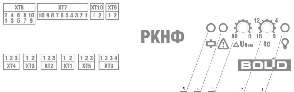
Рисунок 1. Лицевая панель РКНФ
