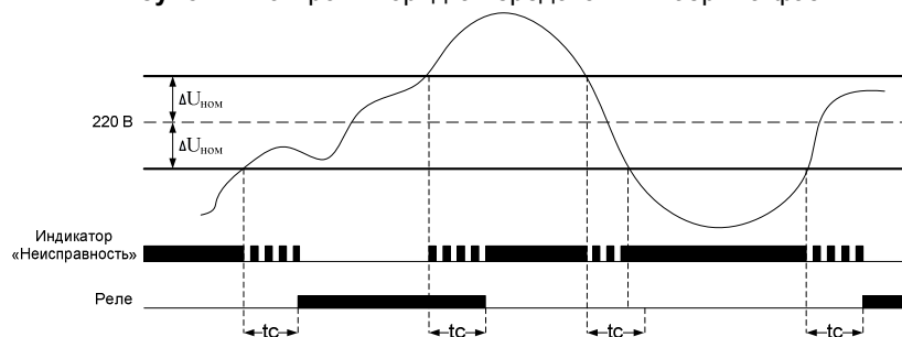
Рисунок 3. Контроль напряжения фазы
