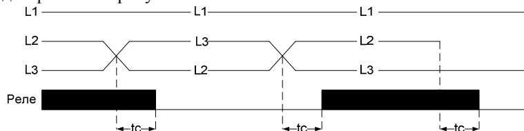
Рисунок 2. Контроль порядка чередования и обрыва фаз
