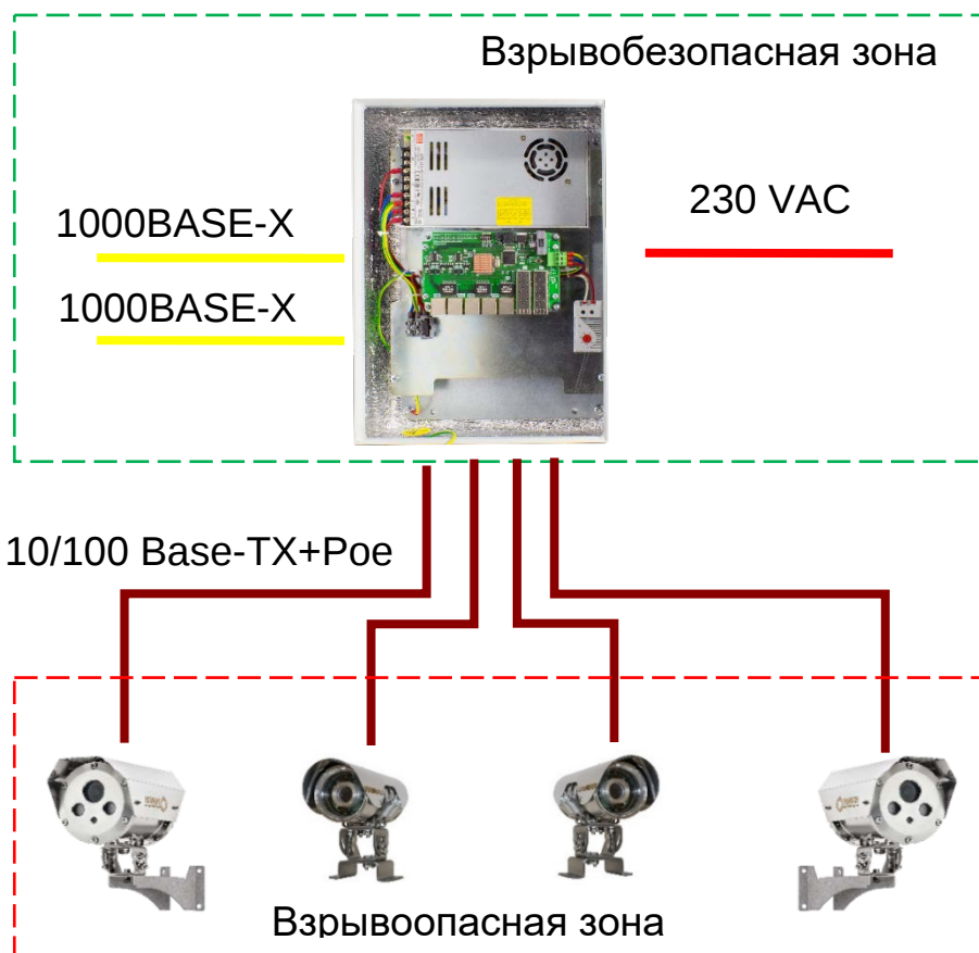
Рисунок 3. Типовая схемы подключения коммутатора по двум оптическим кабелям для работы с взрывозащищенным оборудованием
