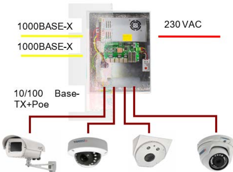
Рисунок 1. Типовая схема подключения коммутатора по одному оптическому кабелю.
