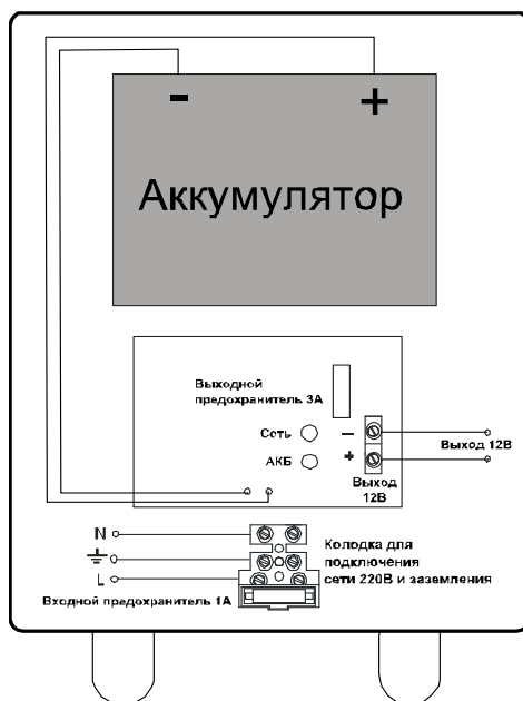
Схема подключения рис. 1
