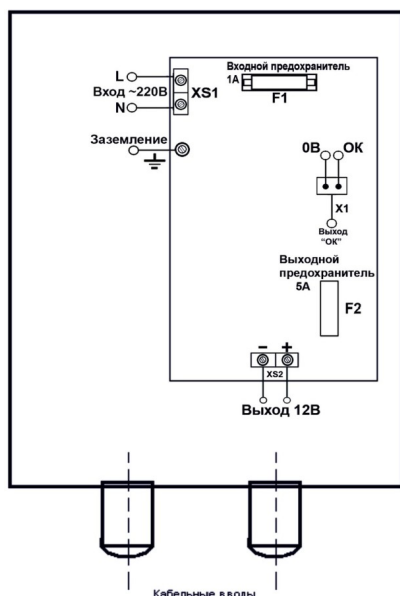
Схема подключения рис. 1
