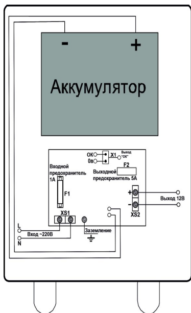
Схема подключения рис. 1
