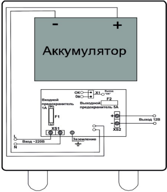
Крепление на DIN-рейку (рис.2)
