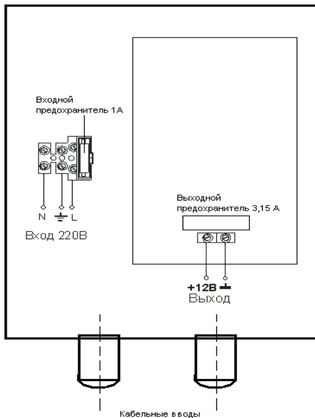
Схема подключения источника согласно рис. 1
