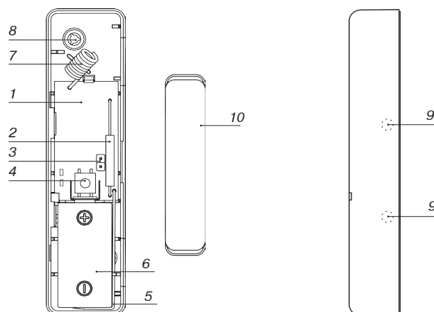
Рисунок 1 – Конструкция «Ri-DO-1»
