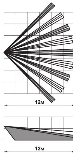
Рисунок 1 – Диаграмма зоны обнаружения
