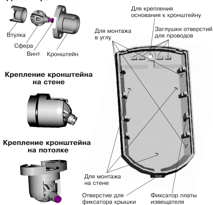
Рисунок 2 – Основание извещателя и кронштейн
