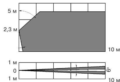
Рисунок 1 – Диаграмма зоны обнаружения
