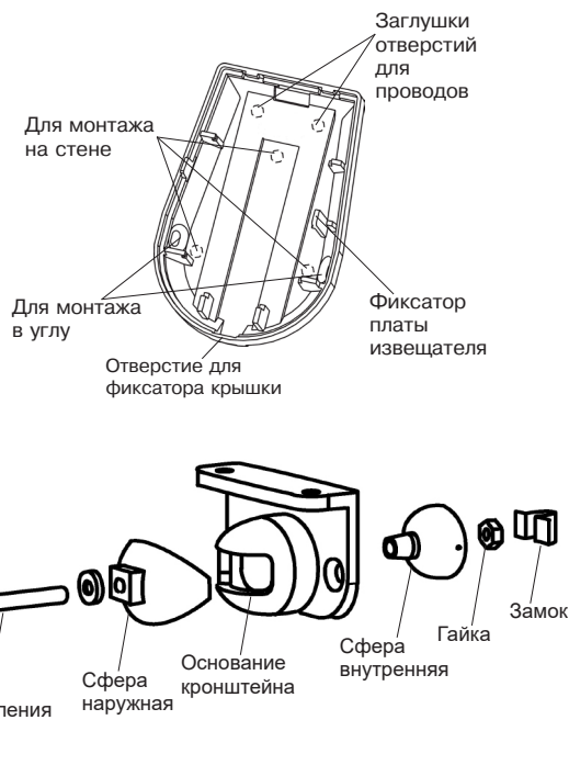
Рисунок 2 – Основание извещателя и кронштейн
