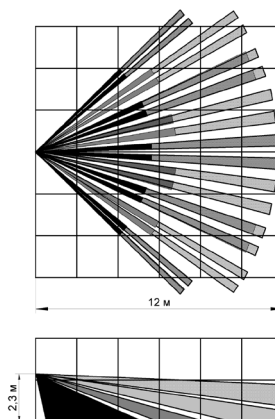
Рисунок 1 – Диаграмма зоны обнаружения извещателя
