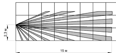
Рисунок 1 – Диаграмма зоны обнаружения извещателя
