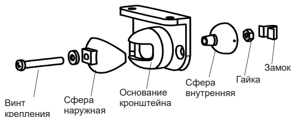
Рисунок 3 – Детали кронштейна
