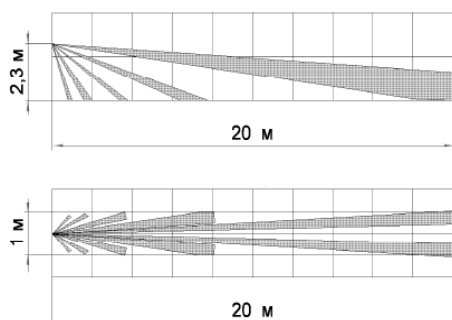
Рисунок 1 – Диаграмма зоны обнаружения
