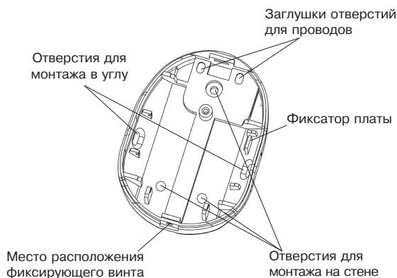
Рисунок 2 – Основание извещателя
