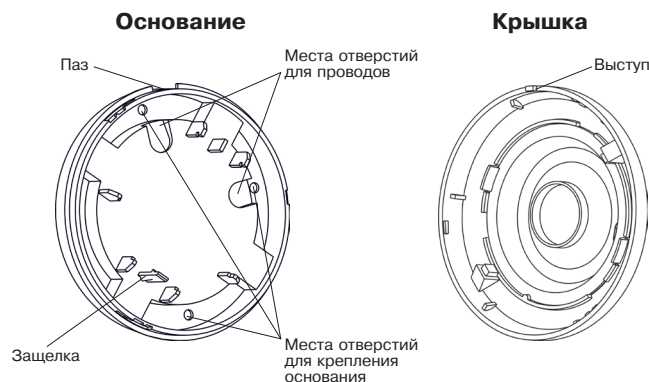
Рисунок 2 – Основание и крышка извещателя
