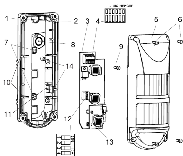
Рисунок 2 – Конструкция извещателя
