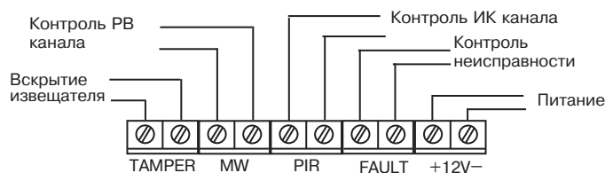
Рисунок 3 – Клеммы подключения
