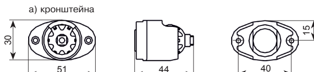
Рисунок 3 – Конструкция извещателя
