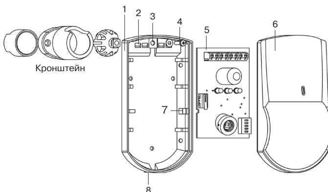
Рисунок 3 – Конструкция извещателя
