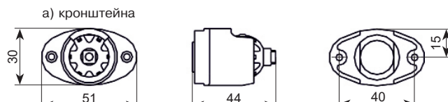
Рисунок 3 – Конструкция извещателя
