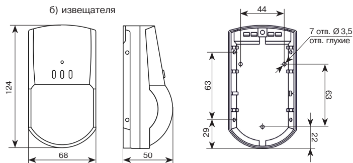
Рисунок 4 – Габаритно-установочные размеры
