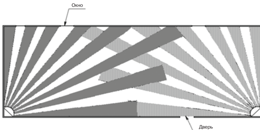
Рисунок В.2 – Установка извещателей «Орлан» и «Орлан-Д» в углу (помещение длиной более 12 м для извещателя «Орлан»; 10 или 8 м для извещателя «Орлан-Д»)
