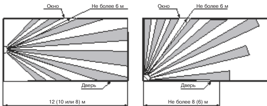
Рисунок В.1 – Установка извещателей «Орлан» и «Орлан-Д» на стене и в углу помещения (длина помещения не более 12 м для извещателя «Орлан»; 10 или 8 м для извещателя «Орлан-Д»)
