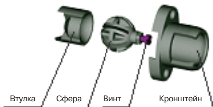
Рисунок Б.1 – Установка извещателя на кронштейне
