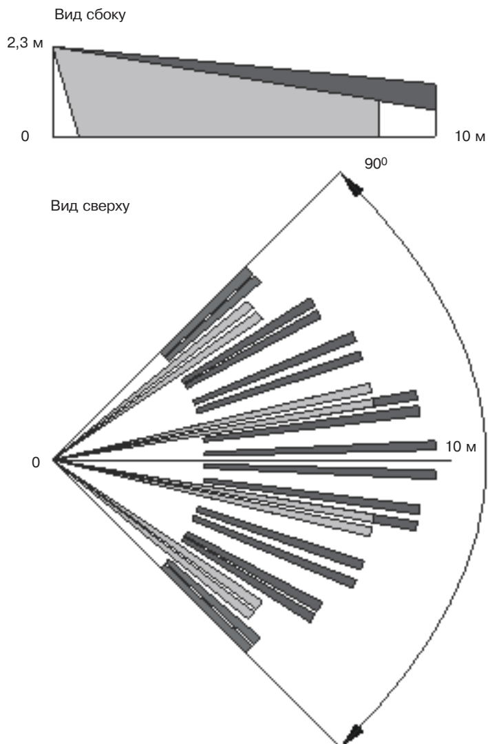
Рисунок А.3 – Структура зоны обнаружения ИК канала извещателя «Орлан-Д»
