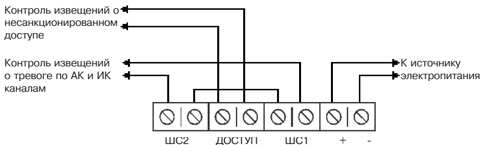
Рисунок Г.2 - Схема подключения извещателя при передаче извещений о тревоге по ИК и АК каналам по отдельному шлейфу сигнализации
