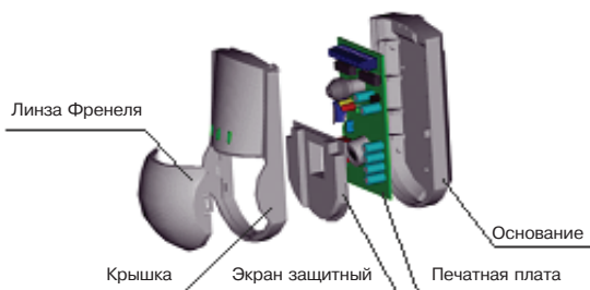
Рисунок Б.5 – Составные части извещателя
