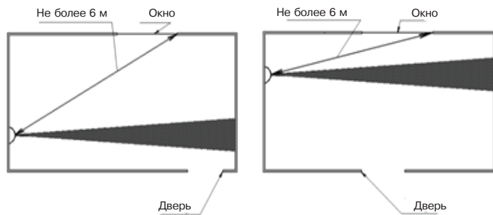
Рисунок В.3 – Установка извещателя «Орлан-Ш» в помещении длиной не более 10 м
