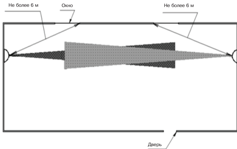
Рисунок В.4 – Установка извещателя «Орлан-Ш» в помещении длиной более 10 м
