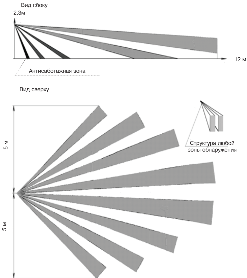
Рисунок А.1 – Структура зоны обнаружения ИК канала извещателя «Орлан»
