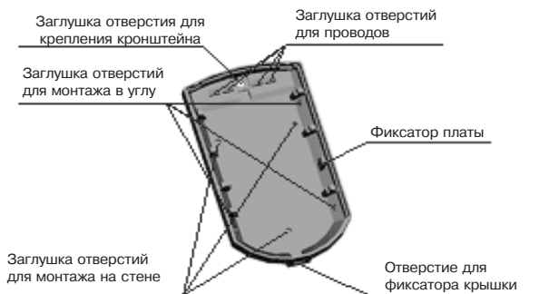
Рисунок Б.6 – Основание извещателя
