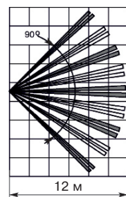
Рисунок 1 – Диаграмма зоны обнаружения ИК канала
