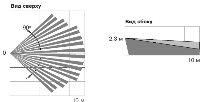
Рисунок 1 – Диаграмма зоны обнаружения
