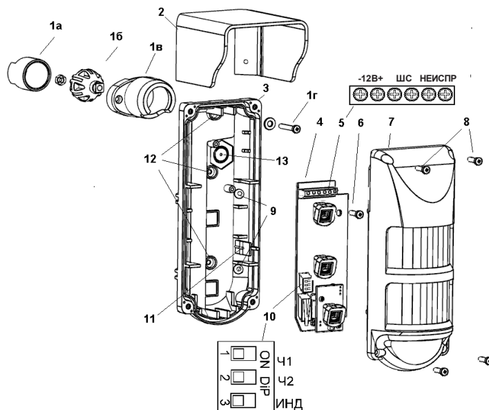
Рисунок 1 – Конструкция извещателя
