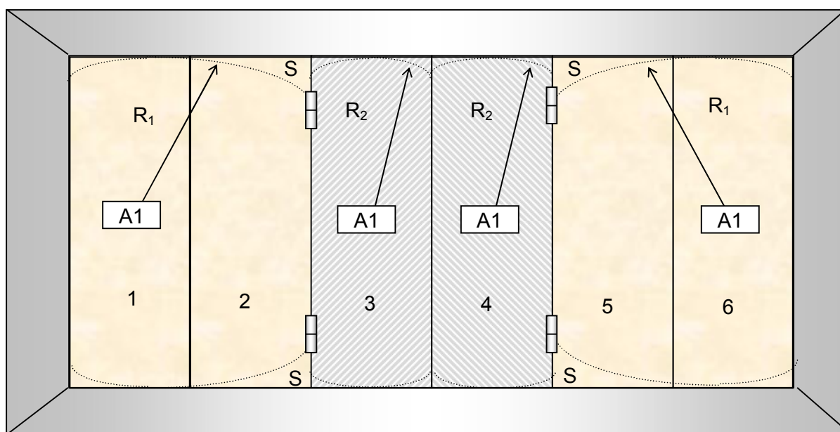
Рисунок В.3 – Установка извещателя с охватом смежной строительной конструкции
