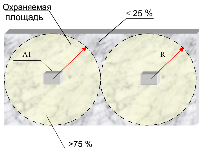
Варианты размещения извещателя на охраняемых конструкциях
