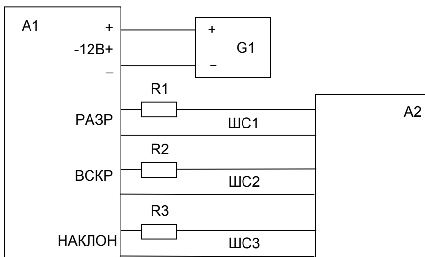
Рисунок Д.1 – Схема подключения извещателя с объединенным «ШС» для передачи извещений "Разрушение", "Наклон", "Вскрытие/отрыв"
