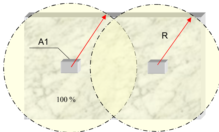
Рисунок В.1 – Установка извещателя на монолитной конструкции с охватом не менее 75 % охраняемой поверхности
