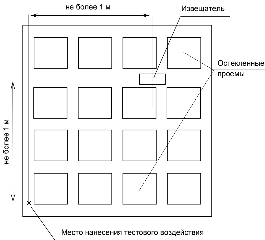
Рисунок В.6 – Установка извещателя на переплете оконной деревянной рамы
