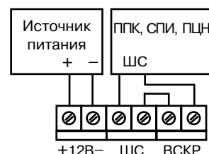
Рисунок 3 – Схема подключения извещателя с объединенными шлейфами сигнализации и вскрытия корпуса
