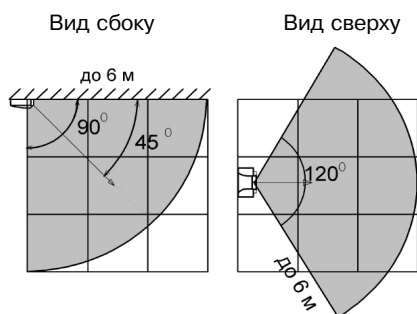
Рисунок 1 - Диаграмма зоны обнаружения АК-канала
