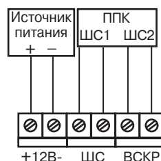
Рисунок 2 – Схема подключения извещателя с отдельными шлейфами сигнализации и вскрытия корпуса
