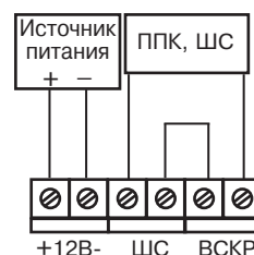
Рисунок 3 – Схема подключения извещателя с объединенными шлейфами сигнализации и вскрытия корпуса
