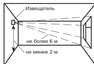
Рисунок 7 – Установка извещателя на противоположной стене
