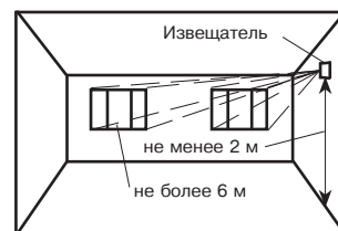
Рисунок 6 – Установка извещателя на боковой стене
