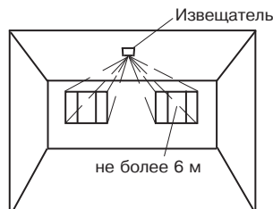
Рисунок 3 – Установка извещателя на потолке
