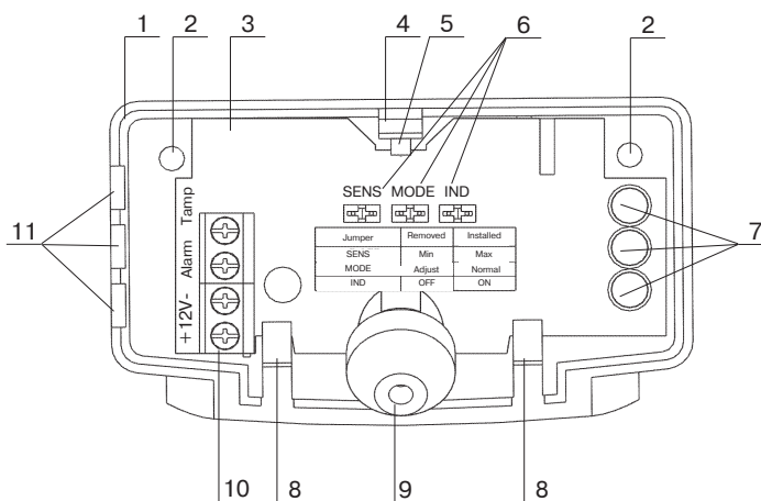
Рисунок 2 — Извещатель со снятой крышкой
