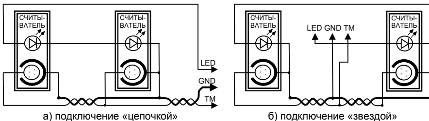
Рисунок 13 – Подключение двух считывателей
