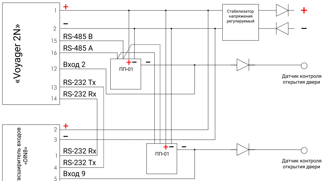
Рисунок 79. Подключение датчика пассажиропотока ПП-01
