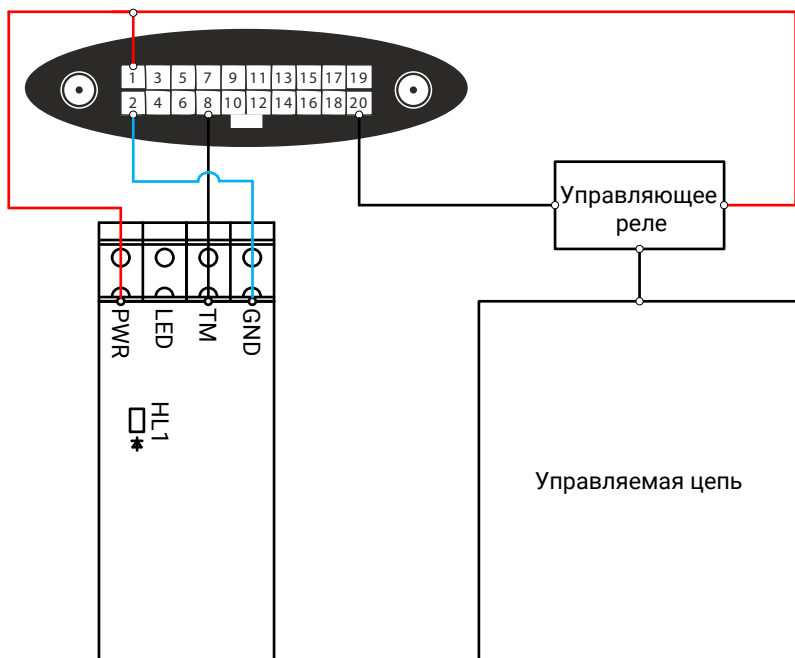
Рисунок 88. Схема подключения блокируемой цепи
