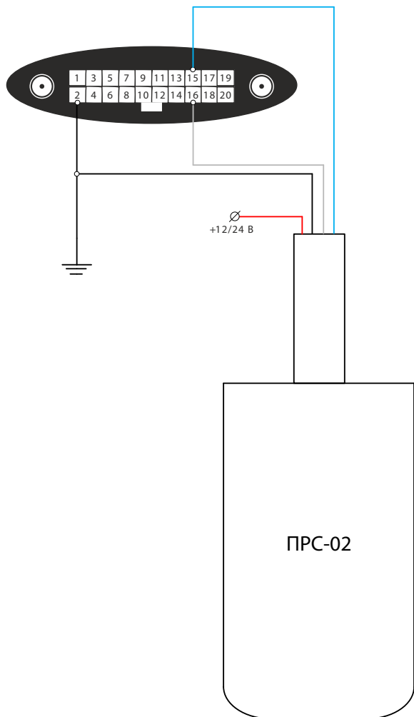
Рисунок 63. Схема подключения датчика контроля работы экскаватора
